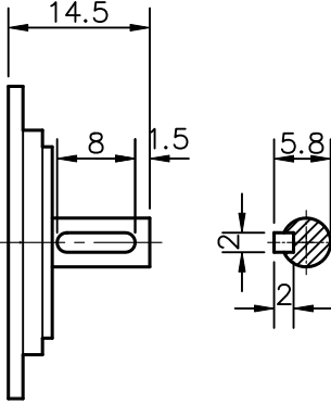
輸入軸 A (標準型)
