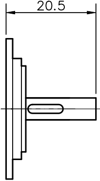
輸入軸 B (加長型)
