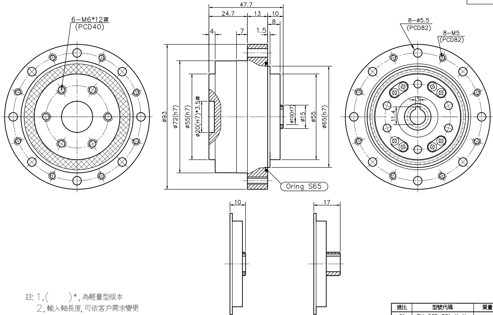
輸入軸 A (標準型)
