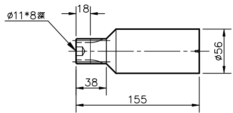
輸入軸 (標準型 A)
