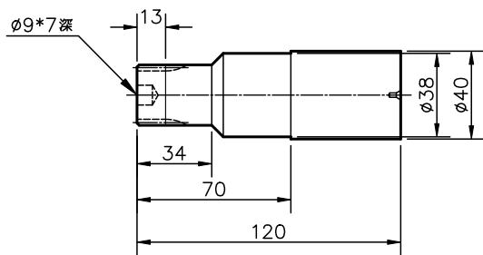
輸入軸
